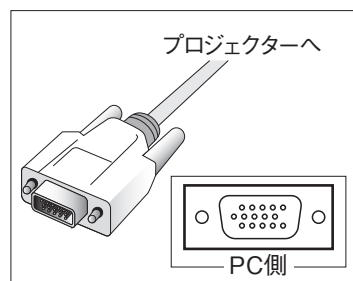
〔mini D-sub 15ピン〕コネクタ形状
