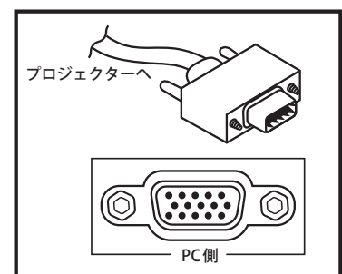
[mini D-sub 15 pin] コネクタ形状
